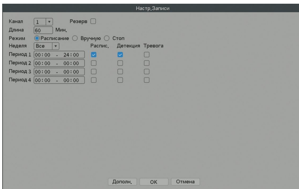
Рис.4.7 Настройка
