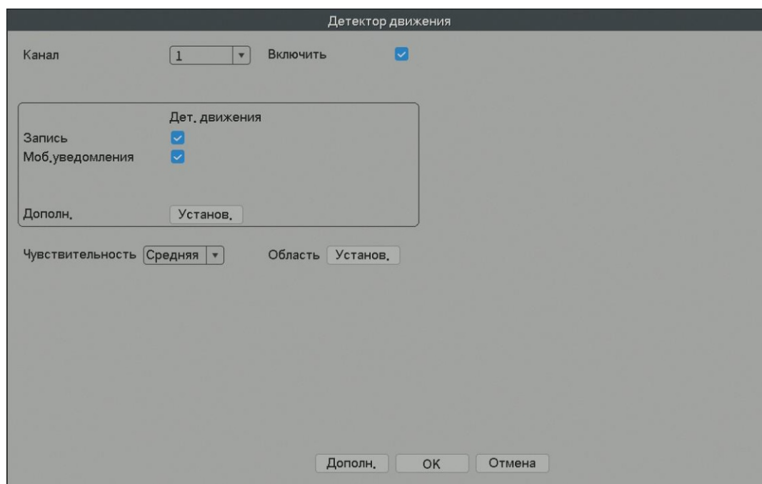
Рис.4 Обнаружение движения
