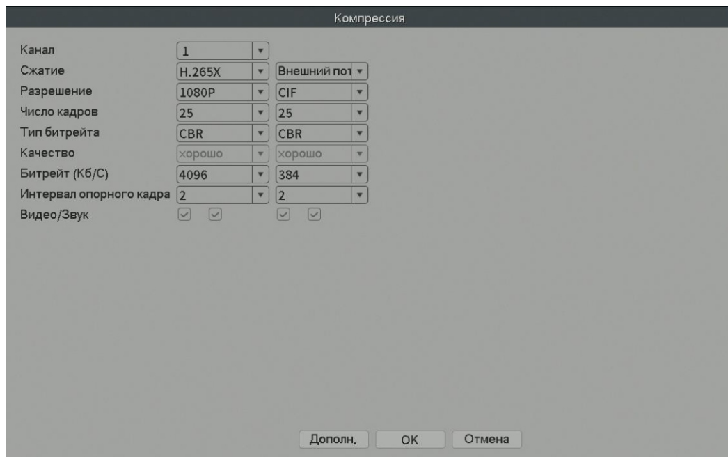
Рис.4.37 Компрессия
