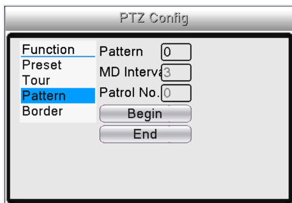
Рис.3.10 Настройки сканирования
