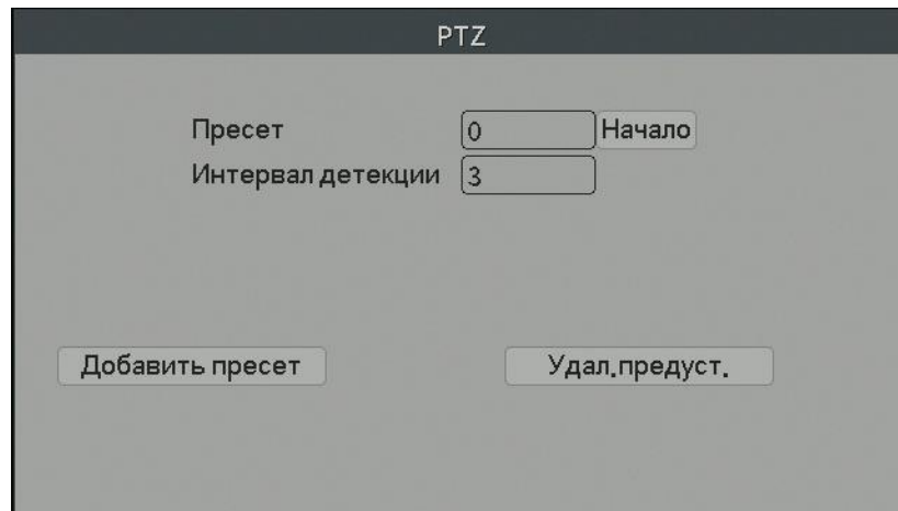
Рис.3.7 Предустановки
