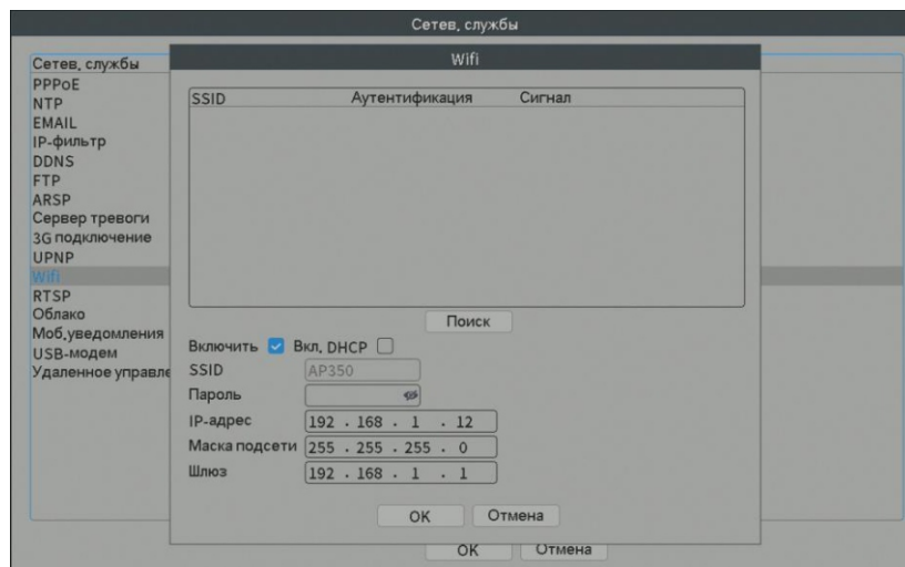
Рис.4.32 Wi-Fi
