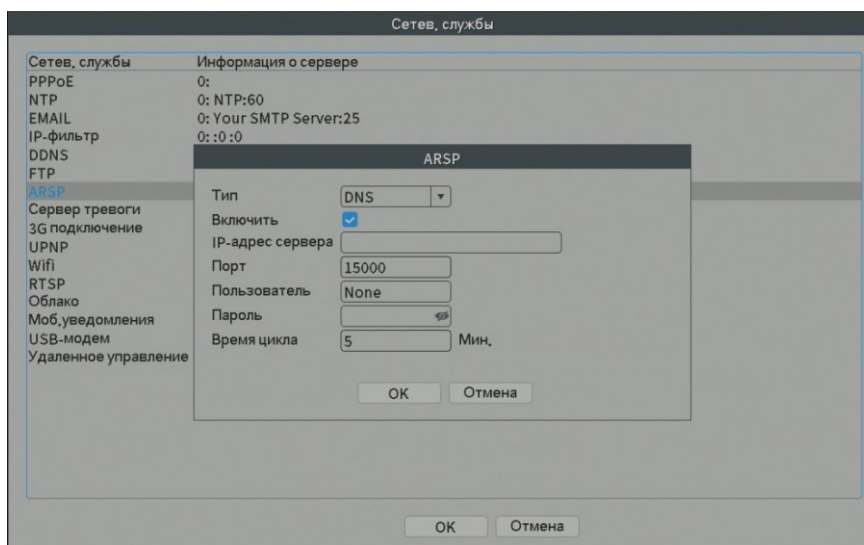
Рис.4.28 ARSP-сервер
