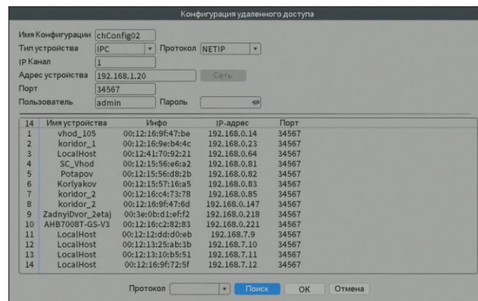
Рис.4.10 Интерфейс удаленной настройки канала
