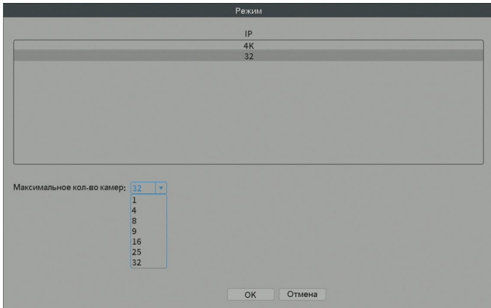
Рис.4.15 Режимы
