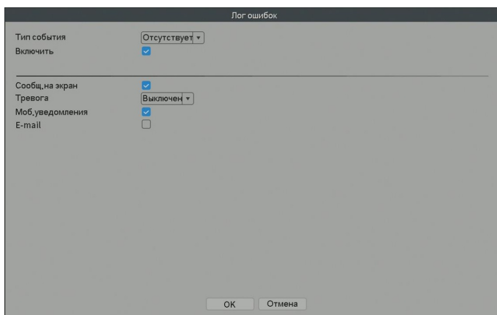
Рис.4.6 Ошибки системы
