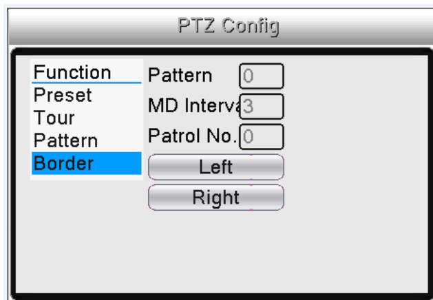
Рис.3.11 Настройки сканирования
