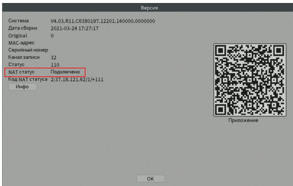
Рис.5.2 Успешное подключение
