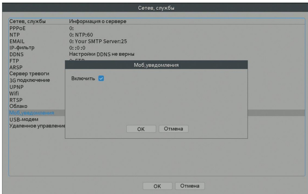
Рис.4.35 Мобильные уведомления
