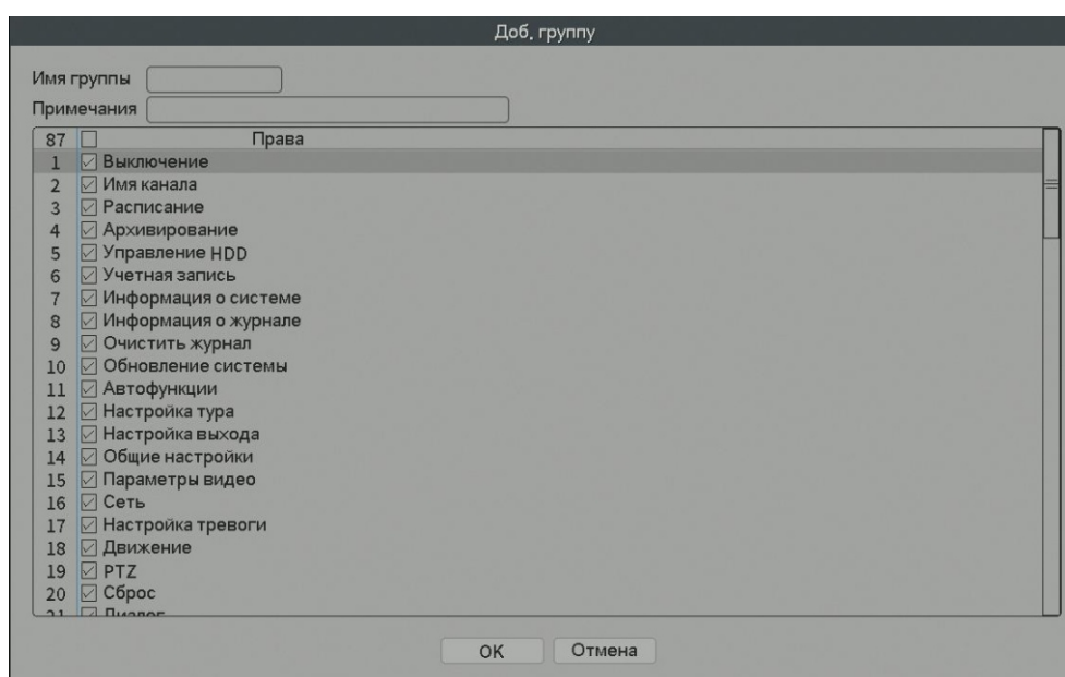
Рис.4.46 Добавление группы
