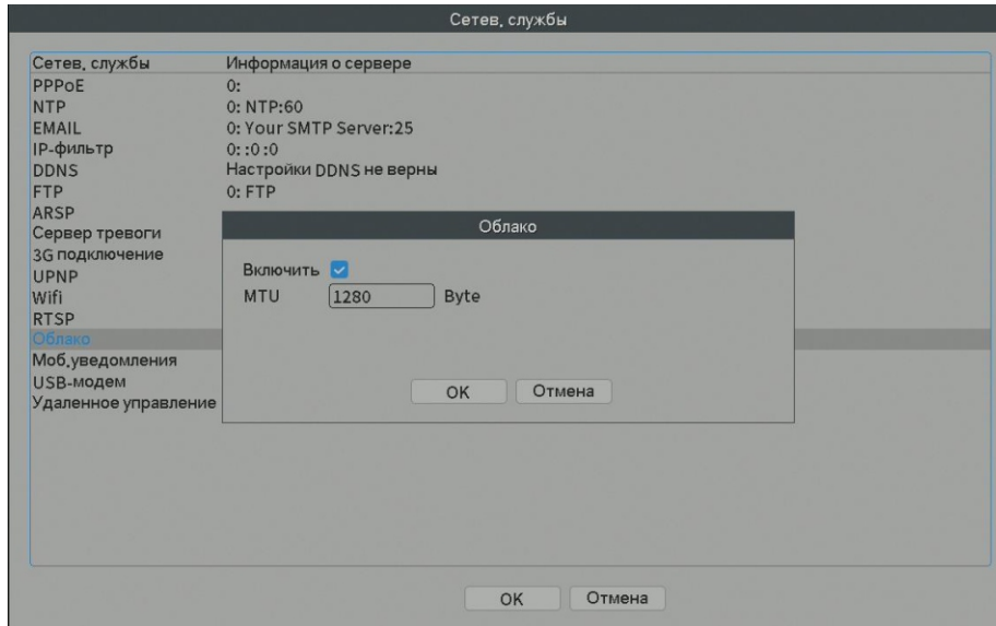
Рис.4.34 «Облако»
