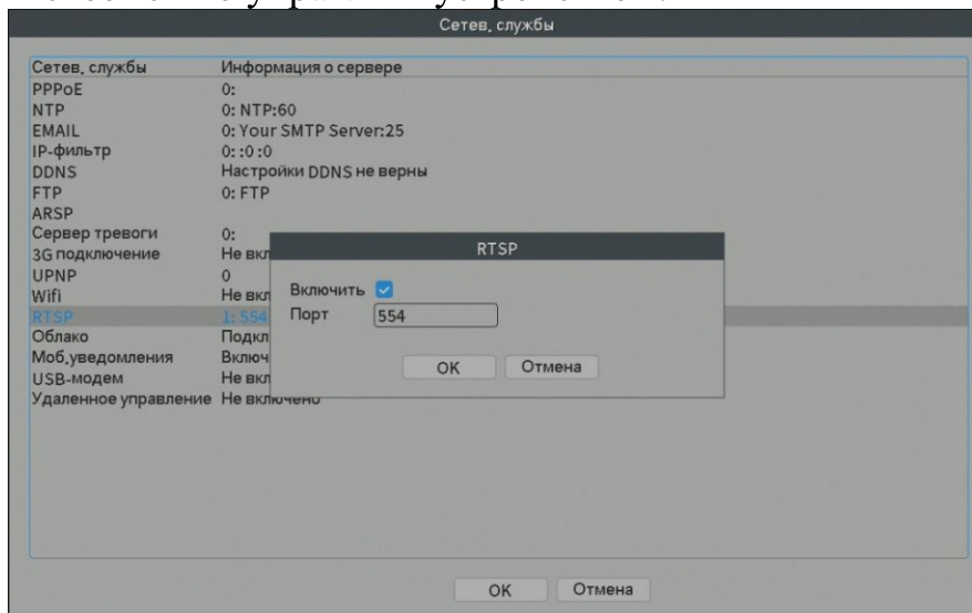
Рис.4.33 RTSP протокол
