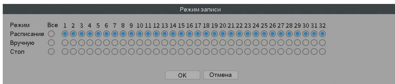
Рис.3.17 Запись
