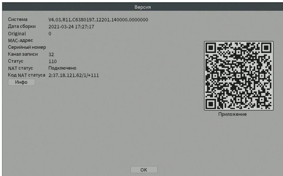
Рис.4.19 Версия
