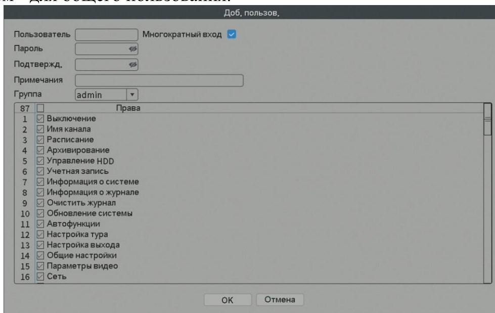
Рис.4.45 Добавление пользователя
